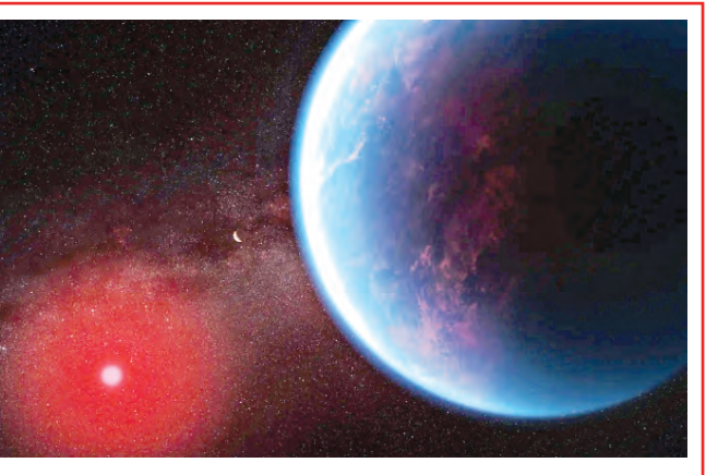
తక్కువ పరిమాణంలో చల్లని ఎరుపు మరగజ్జగా ఉన్నాయి. 2019లో హబుల్ అంతరిక్ష టెలిస్కోప్ దాని వాతావరణంలో నీటి అవిరిని గుర్తించి నవ్వుడు శాస్త్రవేత్తలు దీనిని సౌర వ్యవస్థకు మించిన 'అత్యంత నివాసయోగ్యమైన ప్రపంచంగా' ప్రకటించారు. 2023లో మధుసూదన్ బృందం తమ పరి పరిశీలనలో నీటి సంతృప్తి మిథేన్ అని తేల్చింది.
